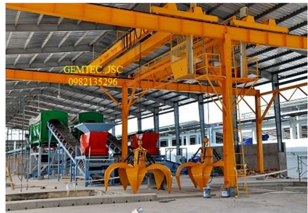
Cầu trục gầu ngoạm
